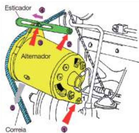
Figura 96 - Forma de esticar a correia
