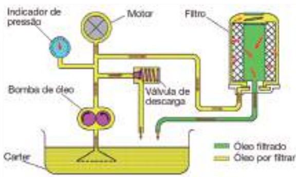
Figura 79 - Filtro de óleo de profundidade com derivação
