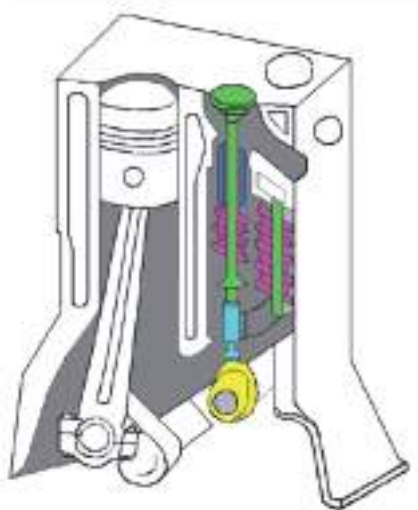
Figura 30 - Válvulas laterais
