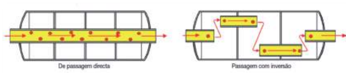
Figura 109 - Silencioso
