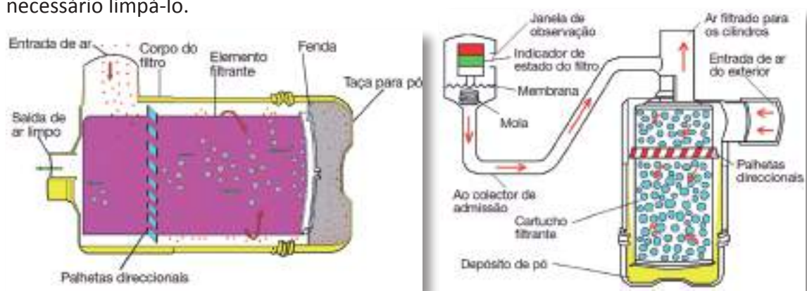
Figura 67 - Filtro com alhetas inclinadas Figura 68 - Filtro com indicador de obstrução
