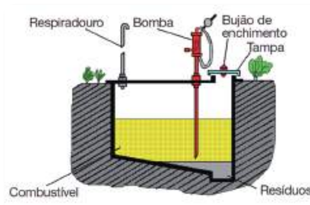
Figura 34 - Armazenamento subterrâneo
