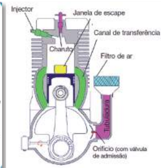
Figura 6 - Motor 2 tempos de combustão
