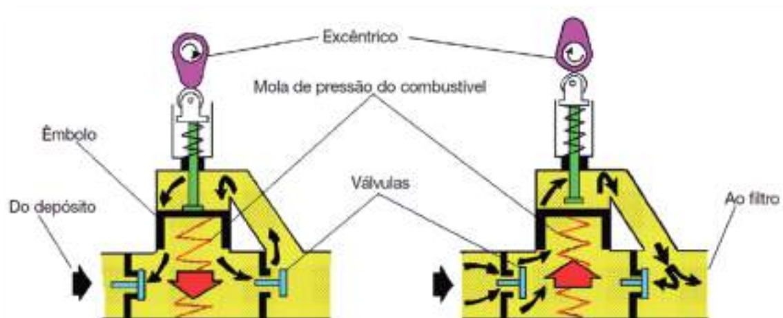
Figura 43 - Bomba de pistão
