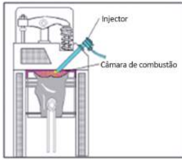
Figura 61 - Injeção direta
