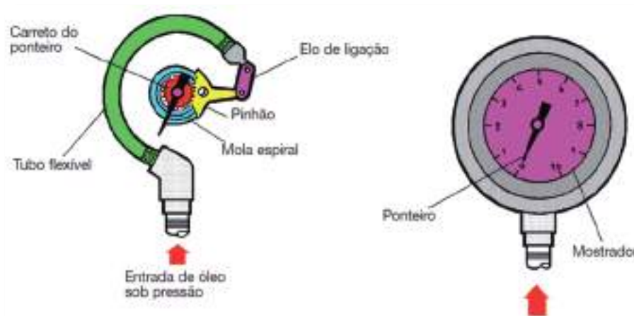
Figura 85 - Manómetro mecânico
