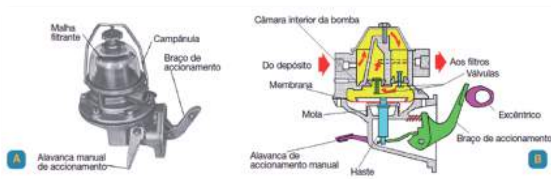
Figura 41 - Bomba de diafragma
