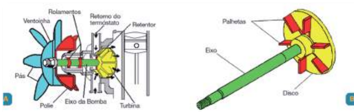
Figura 97 - Bomba de água
