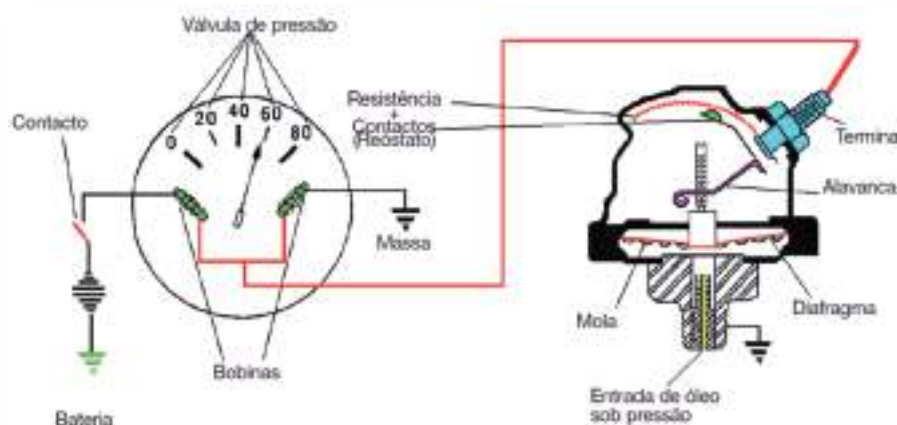
Figura 86 - Manómetro elétrico
