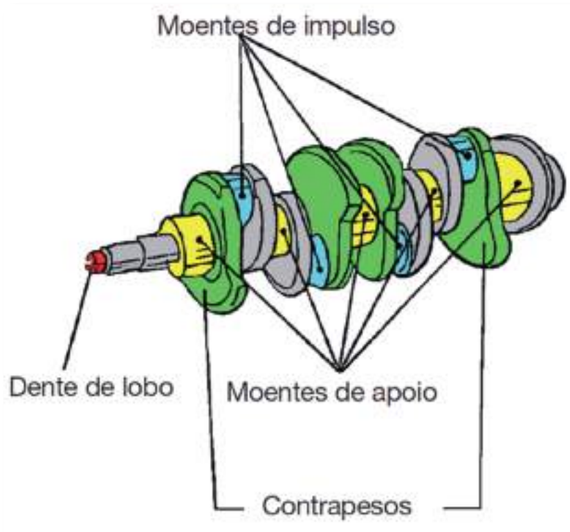
Figura 17 - Cambota
