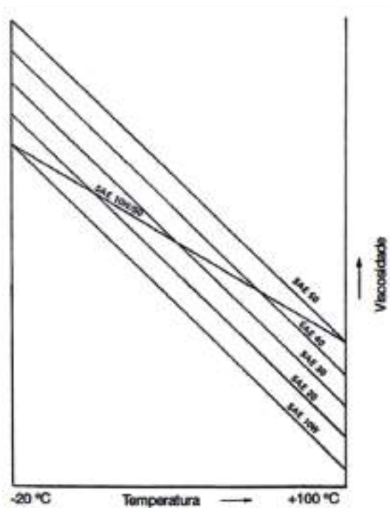
Figura 88b - Monograduados versus Multigraduados
