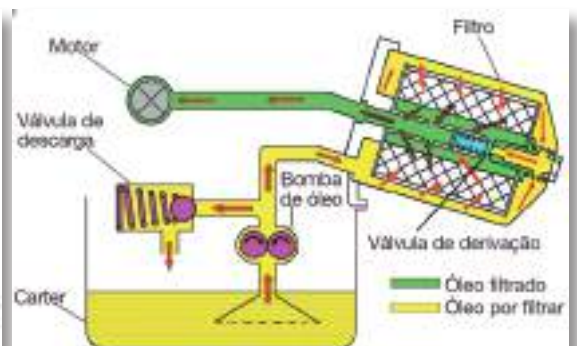
Figura 80 - Filtro de óleo de profundidade de filtragem total
