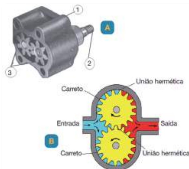
Figura 76: 1 - Corpo da bomba 2 - Eixo de acionamento 3 - Carretos Normalmente, à entrada da
