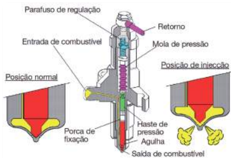
Figura 53 - Injetor
