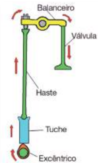
Figura 28 - Haste
