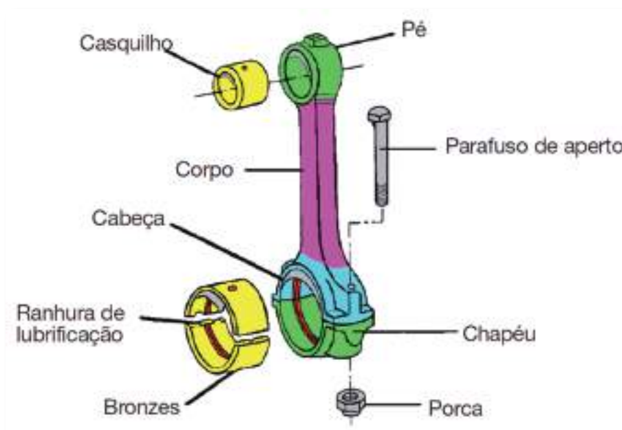
Figura 16 - Biela
